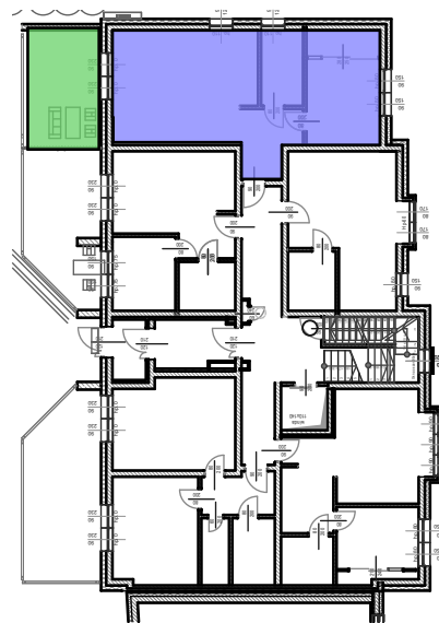
RZUT PARTERU
